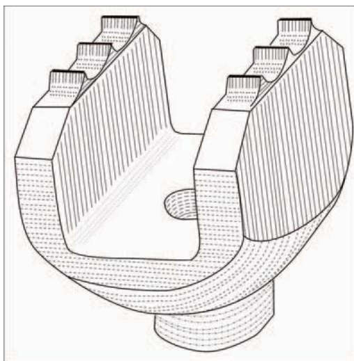
Rys. 3.10. Koronka wielozębna udarowa (wg Albowa 1975)
