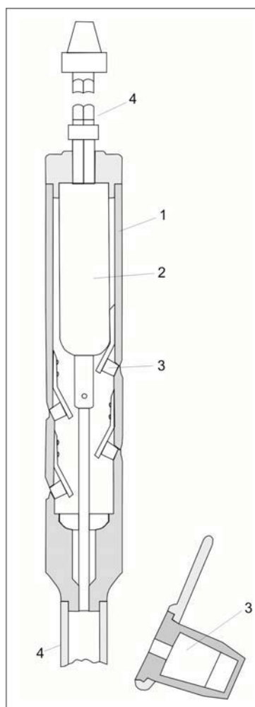
Rys. 2.2. Boczny próbnik sprężynowy dla kilku próbek
