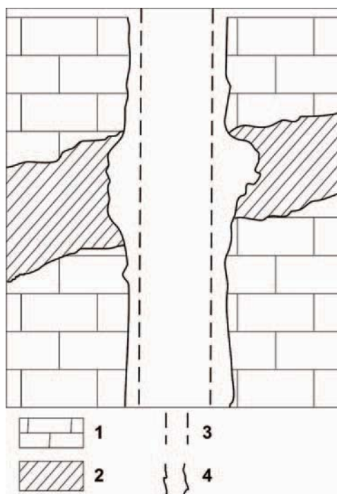
Rys. 3.5. Przykład deformacji założonego kształtu bruzdy wskutek selektywnego wykruszania minerałów o małej wytrzymałości (np. galeny w złożach rud Zn – Pb) 1 – wapień, 2 – żyła kruszcowa (galena), 3 – założony kształt bruzdy, 4 – kształt rzeczywisty
