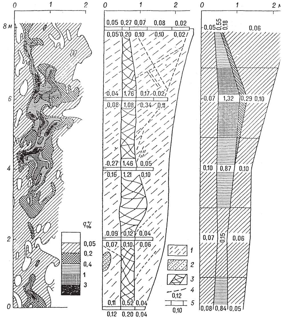
Rys. 8.1. Zróżnicowanie zawartości składnika użytecznego (Sn) w złożu (A.P. Oczkur 1985) a – na podstawie opróbowania punktowego, b – uśrednione w próbkach brzdowych, c – uśrednione w blokach. 1 – iłowce, 2 – piaskowce, 3 – brekcje, 4 – drobne uskoki, 5 – zawartości: w górze na podstawie oznaczeń rentgenofluorescencyjnych, w dole na podstawie próbek brzdowych)
