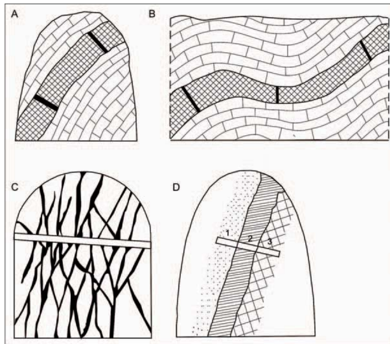
Rys. 3.7. Pobieranie próbek bruzdowych w wyrobiskach górniczych A, B – w złożu pokładowym lub żyłowym, C – w złożu sztokwerkowym, D – w złożu żyłowym o niejednorodnej budowie, 1, 2, 3 – próbki odcinkowe
