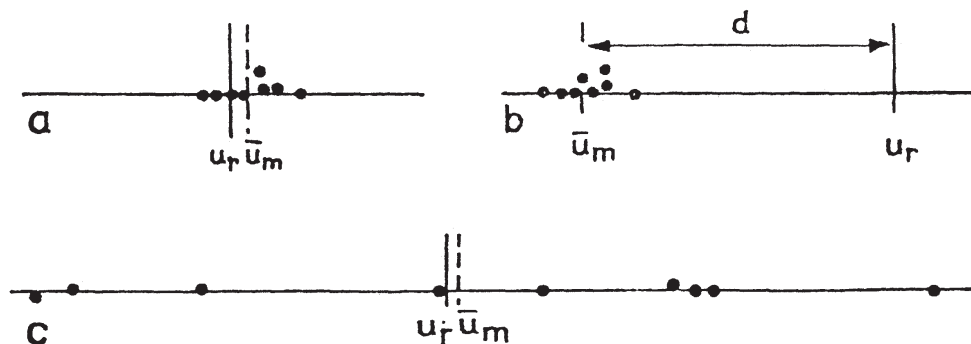
Rys. 7.2. Dokładność pomiaru
